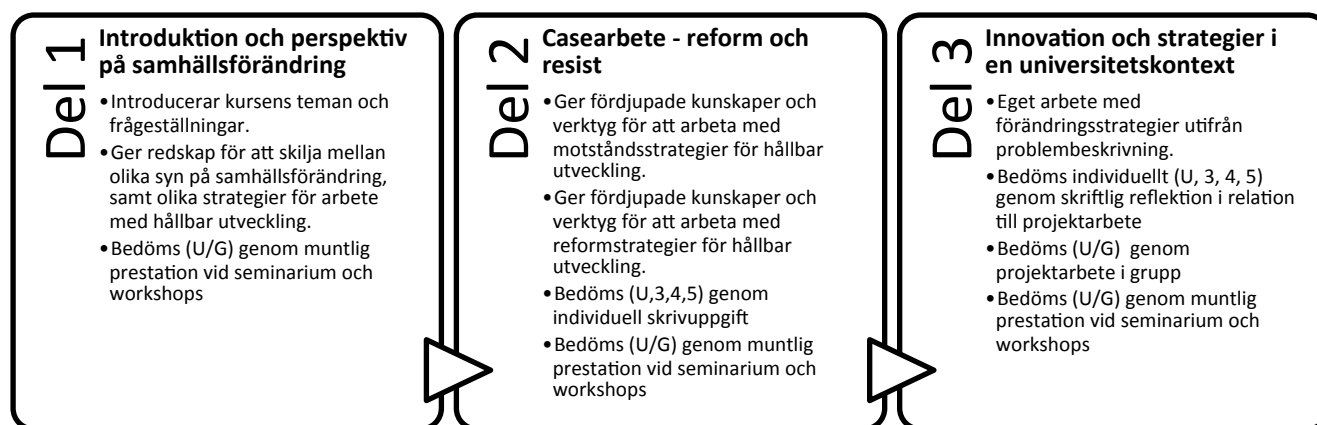
Figur 1: Kursens grovstruktur.
